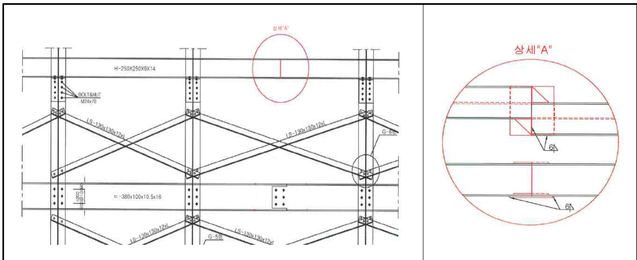
[그림 1] 강관버팀보 종방향 받침부재 연결부 시공상세도
