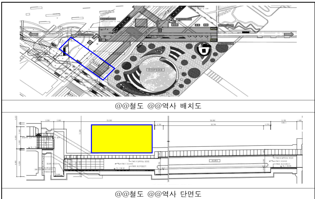
[그림] @@식물원 연결통로 설계 현황
