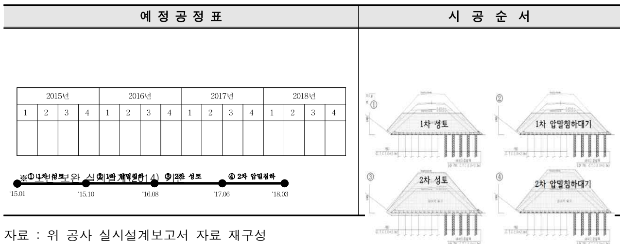
[표 1] 연약지반 시공 예정공정표 및 시공순서
